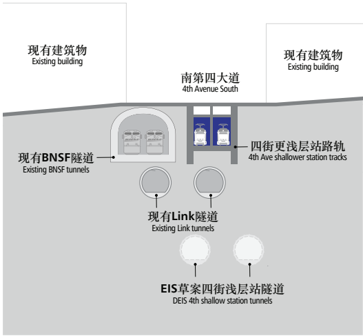
横切图 A Section A
